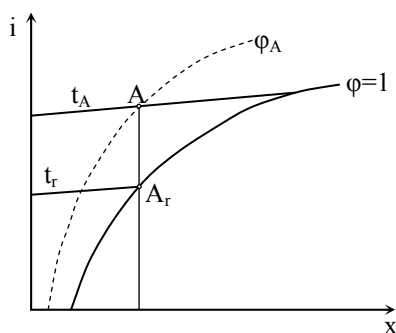
Rys.1. Wyznaczanie wilgotności względnej \varphi na wykresie i-x według wskazań higrometru kondensacyjnego
