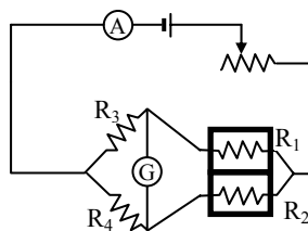
Rys. 3. Schemat higrometru opartego na zasadzie zmiany przewodnictwa cieplnego powietrza wilgotnego
