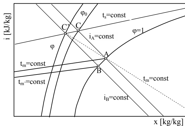
Rys. 8. Wyznaczanie wilgotności względnej wg wskazań psychrometru na wykresie i-x
