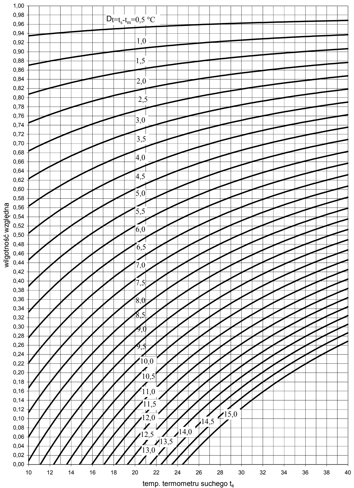
Rys. 9. Wykres psychrometryczny dla v=0,46 \text{ [m/s]}
