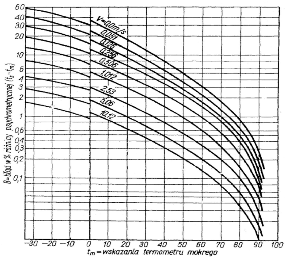
Rys. 11. Wykres błędów dla wskazań psychrometrów
