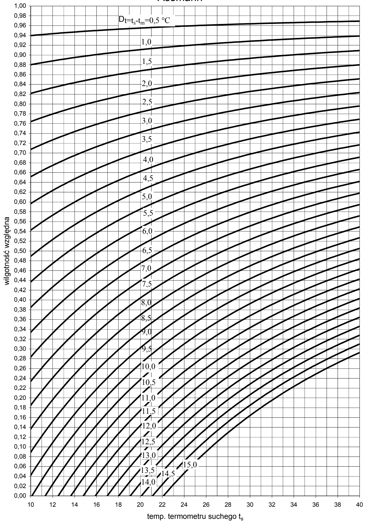
Rys. 10. Wykres psychrometryczny dla v=2,5 [m/s]
